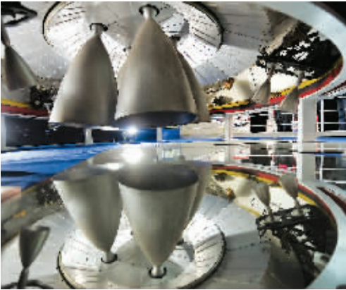
■ 上海制造的“神七”2500N 双元发动机底部
