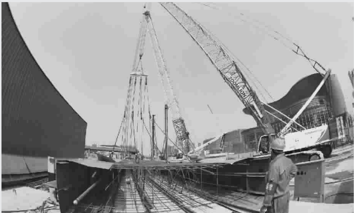
■ 北横通道加快建设,上海隧道的工作人员进行钢筋槽入槽作业
