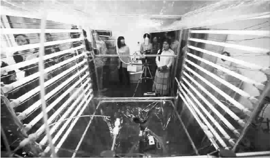
■ 复旦大学用实验装置模拟大气环境,分析 PM2.5 的构成
