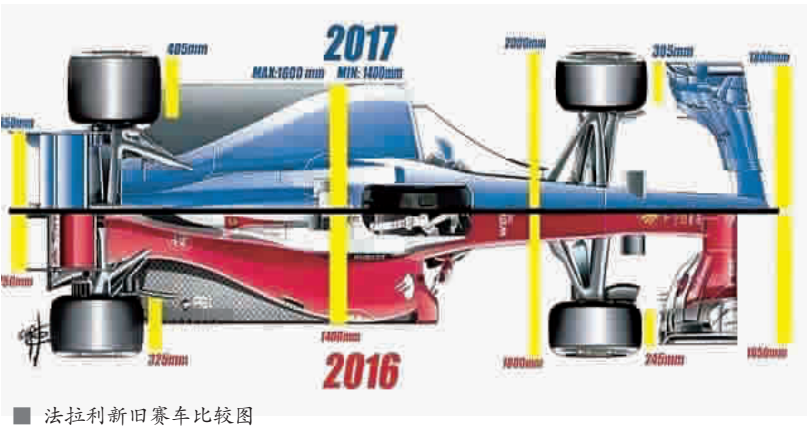
■ 法拉利新旧赛车比较图
