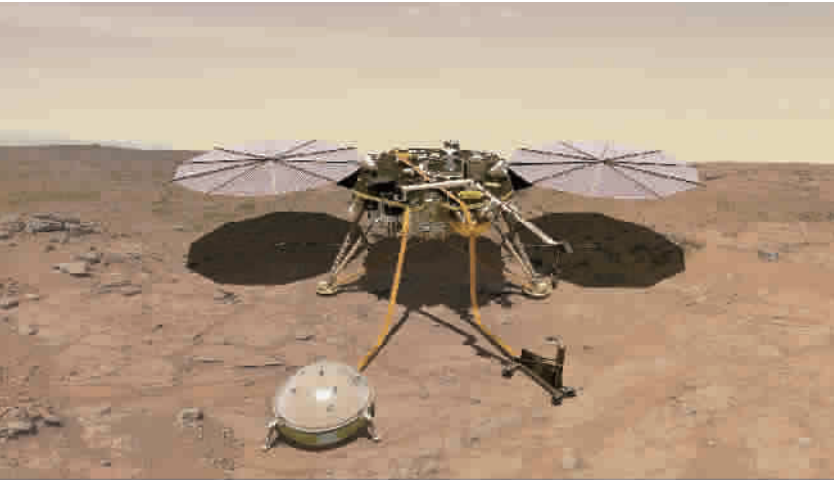
■ “洞察”号在火星着陆后效果图
