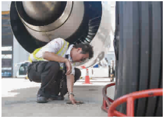
■ 昨天下午,虹桥机场工作人员检查登机桥地锚,确保台风过境期间,航空器与地面固定紧密
